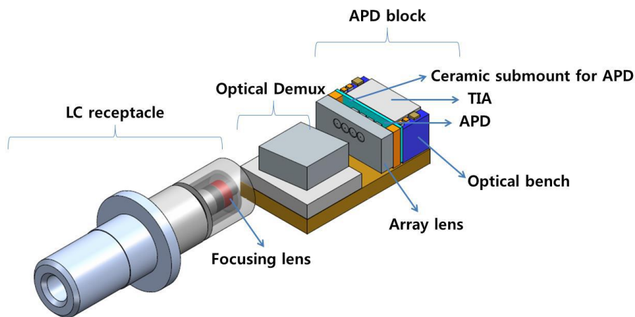
내부 구조
